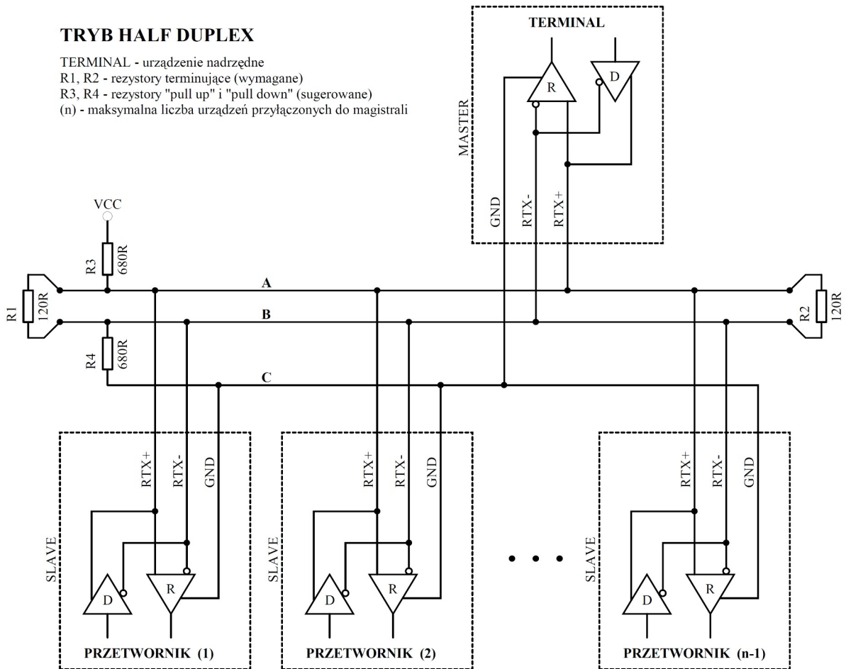
Rysunek 5. Sposób podłączenia przetwornika do magistrali RS-485 pracującej w trybie HALF DUPLEX.
