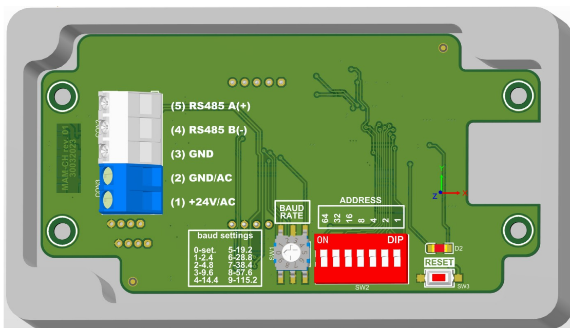
Rysunek1. Widok obwodu drukowanego przetwornika.
