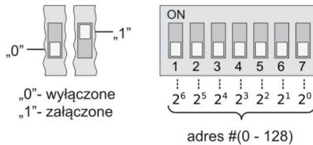
Rysunek 2. Adresacja przetwornika.
