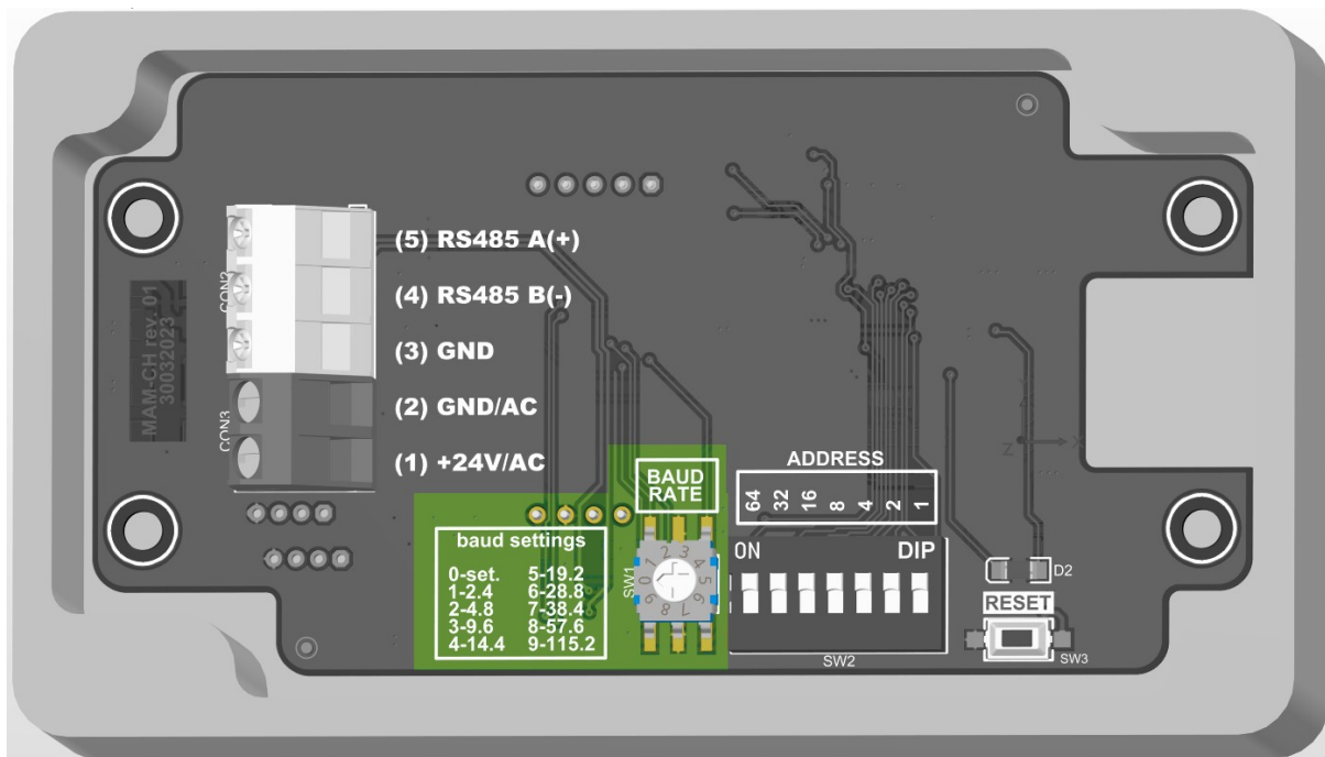
Rysunek 3. Konfiguracja prędkości interfejsu RS-485.
