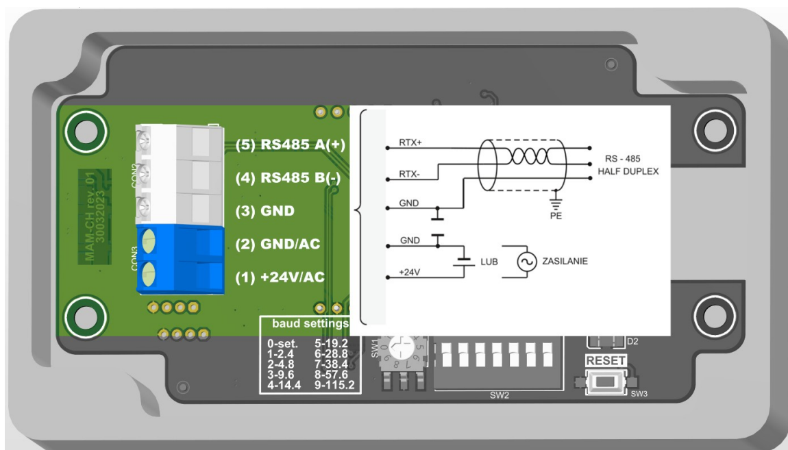
Rysunek 1. Schemat podłączenia przetwornika.
